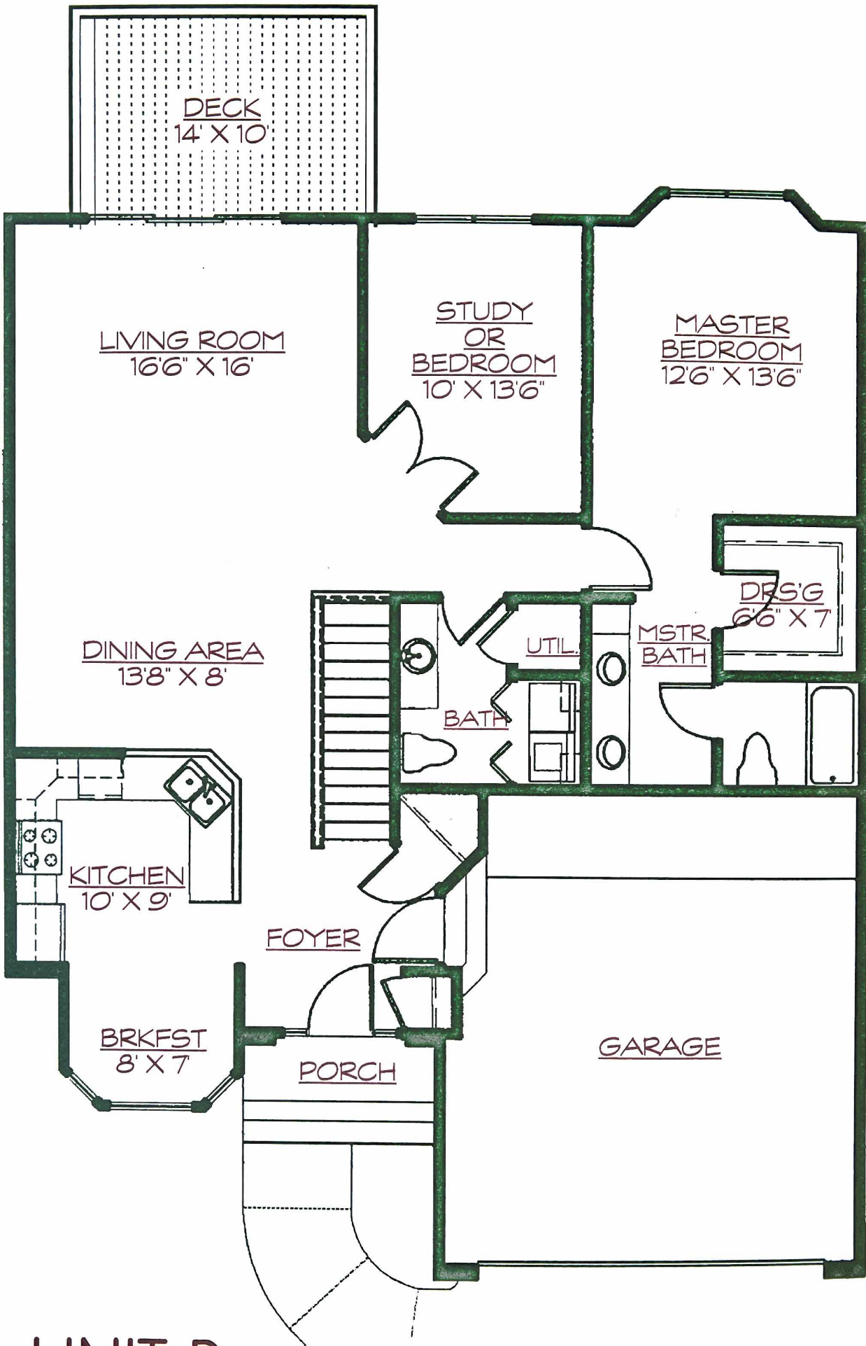
UNIT B (INTERIOR) 1343 S.F.
